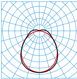
OleveonF 12 L 4000-840 ETDD PC+LLWRC LV TX056116
