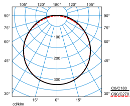
3331 G2 D2 LED2400-830 ETDD +LLWC 01
