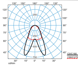
7850 HE+ LDAN40 840 L150 1 50
