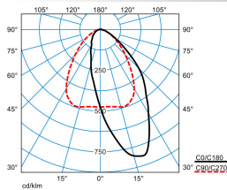
ELINE LAN160 840 L225 1 20
