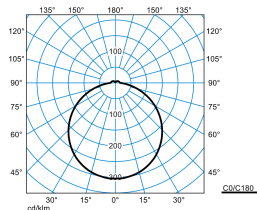
Olisq RWD2 DW 40-830 ET + Olisq RWD2 ZDR 1/2 01 TX426075
