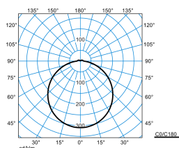
Olisq RWD2 DW 40-830 ET + Olisq RWD2 C 01 TX425803
