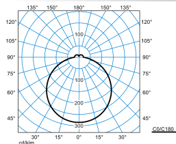
Olisq RWD2 DW 40-830 ET TX375562
