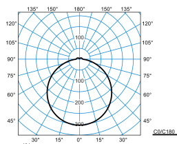
Olisq RWD2 DW 40-830 ET + Olisq RWD2 ZDR 1/2 05 TX428714
