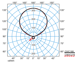
Luceos S-T PAW-IL 300-830 ETDI 03+LLWP (LEO2)
