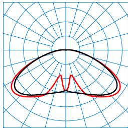
Publisca P1W-RBT-LRA/1500-740 2G1S ET (CLO end value) TX300180 ■ C0 - C180 ■ C90 - C270 DIN 5040: A20 UTE: 0.97 l + 0.03 T DLOR: 97 % ULOR: 3 % CEN Flux Code: 26 63 91 97 100 4 16 28 3
