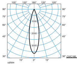
E-Line PRO 78 Lentyp L-MF 40-EW M48 ETBLE 03 Blank
