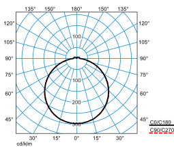
Olisq QWD3 DW 45-830 ET EB3 + Olisq QWD3 ZDR 1/2 03
