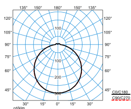
Olisq QWD3 DW 45-830 ET EB3 + Olisq QWD3 ZDR 1/2 01
