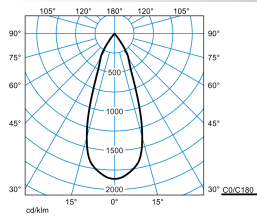
TaroMini 3PTD RF-FL 30-830 M33 ET 01
