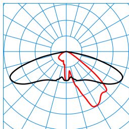
Publisca P1-AB2L-LRA/4200-730 6G1S ET (CLO initial value) TX300191 ■ C0 - C180 ■ C90 - C270 DIN 5040: A30 UTE: 1,00 G DLOR: 100 % ULOR: 0 % CEN Flux Code: 35 74 97 100 100
