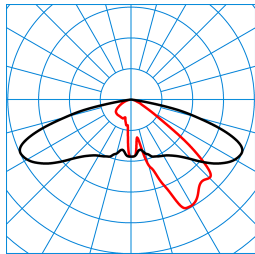
Publisca P1-AB2L-LRA/4200-730 6G1S ET (CLO end value) TX300677 ■ C0 - C180 ■ C90 - C270 DIN 5040: A30 UTE: 1,00 G DLOR: 100 % ULOR: 0 % CEN Flux Code: 35 74 97 100 100
