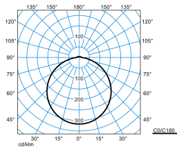
Olisq RWD4 DW 40-840 ET HFS IP54 PC + Olisq RWD4 ZDR 1/2 01
