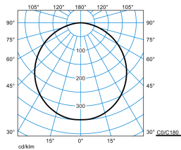
Olisq RWD4 DW 40-840 ET HFS IP54 PC + Olisq RWD4 ZDR 1/1 01
