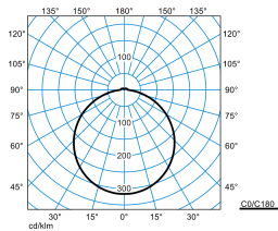
Olisq RWD4 DW 40-840 ET HFS IP54 PC + Olisq RWD4 ZDR 1/2 03
