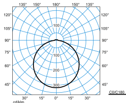
Olisq RWD4 DW 40-840 ET HFS IP54 PC + Olisq RWD4 ZDR 1/2 05
