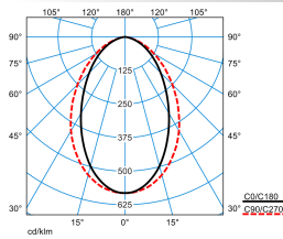
FidescaSD G3 D4 DN 200-865 ETDD TX199974
