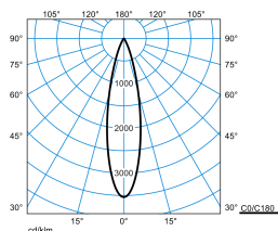
YNSx2LY 7x65 L-MF 01/05 10-940 DD 01 (LEO1)
