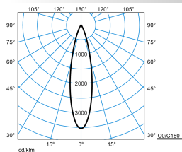
YNSx2LY 7x65 L-MF 01/05 10-940 DD 01 (LEO2)
