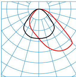
Cultega Act T SMC PAW 600 ETDI KL 05 (ACTDCW) TX770469 ■ C0 - C180 ■ C90 - C270 DIN 5040: A40 UTE: 1,00 D DLOR: 100 % ULOR: 0 % CEN Flux Code: 54 85 97 100 100
