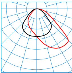
Cultega Act T SMC PAW 600 ETDI KL 05 (ACTDWW) TX770477 ■ C0 - C180 ■ C90 - C270 DIN 5040: A40 UTE: 1,00 D DLOR: 100 % ULOR: 0 % CEN Flux Code: 54 85 97 100 100
