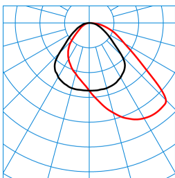
Cultega Act T SMC PAW 600 ETDI KL 05 (ACTDSU) TX770472 ■ C0 - C180 ■ C90 - C270 DIN 5040: A40 UTE: 1,00 D DLOR: 100 % ULOR: 0 % CEN Flux Code: 54 85 97 100 100
