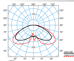
Publisca P1W-RBT-LR/2600-730 3G1S ET (CLO initial value)
