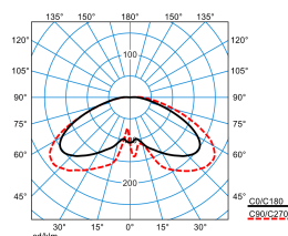
Publisca P1W-RBT-LR/2600-730 3G1S ET (CLO end value)
