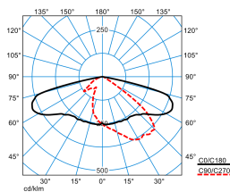
LnPlus 40-AB7L/6200-740 12G1 ETDD (CLO end value)
