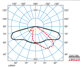
LnPlus 40-AB7L/6200-740 12G1 ETDD (CLO initial value)
