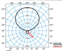
Luceos S BS G3 PAW-IL 125-8TW ETDS FT 01 (DWW)
