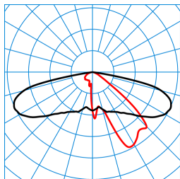
Publisca P1-AB2L-LR/2000-740 3G1S ET (CLO initial value) TX300493 ■ C0 - C180 ■ C90 - C270 DIN 5040: A30 UTE: 1,00 l DLOR: 100 % ULOR: 0 % CEN Flux Code: 34 71 96 100 100
