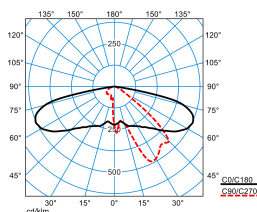
Publisca P1-AB2L-LR/2000-740 3G1S ET (CLO end value) TX301882 DIN 5040: A30 UTE: 1,00 l DLOR: 100 % ULOR: 0 % CEN Flux Code: 34 71 96 100 100
