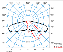
Publisca P1-AB2L-LR/2000-740 3G1S TX047518 DIN 5040: A30 UTE: 1,00 l DLOR: 100 % ULOR: 0 % CEN Flux Code: 34 71 96 100 100
