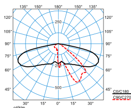
Publisca P1-AB2L-LR/2000-740 3G1S ET (CLO initial value) TX300493 DIN 5040: A30 UTE: 1,00 l DLOR: 100 % ULOR: 0 % CEN Flux Code: 34 71 96 100 100
