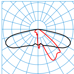
Publisca P1-AB2L-LR/2000-740 3G1S ET (CLO end value) TX301882 ■ C0 - C180 ■ C90 - C270 DIN 5040: A30 UTE: 1,00 l DLOR: 100 % ULOR: 0 % CEN Flux Code: 34 71 96 100 100
