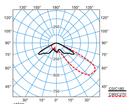
LnPlus 40-AM19L-SLR1/2200-722 2G1 ET (CLO initial value) TX377409
