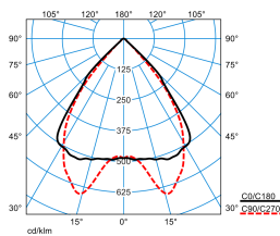
SFlow C1-L MRX LED3200-840 ET 01 TX721277
