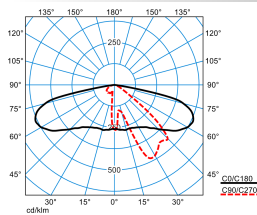
Publisca P2-AB2L/1500-740 2G1S
