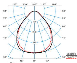
ArimoFit M73 PW19 30-840 ET + ArimoFit Sky M73-TS ZER
