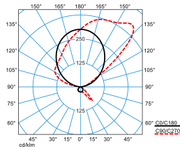
Luceos S G3 PAW-IA 170-930 ETDS FT 03
