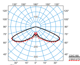
Publisca P1-RB6L-LR/3200-740 4G1S ET (CLO initial value)
