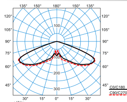
Publisca P1-RB6L-LR/3200-740 4G1S
