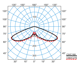
Publisca P1-RB6L-LR/3200-740 4G1S ET (CLO end value)
