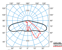
Publisca P1-AB2L-LR/1200-740 2G1S ET (CLO end value) TX300499 DIN 5040: A30 UTE: 1,00 G DLOR: 100 % ULOR: 0 % CEN Flux Code: 34 70 96 100 100
