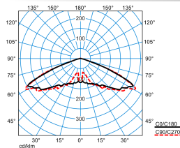
Publisca P1W-RB6L/1500-740 2G1S TX053510
