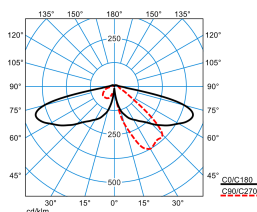
8841LS-UE 260-AB2L/1500-730 3G2 ET (CLO end value)
