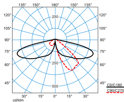
8841LS-UE 260-AB2L/1500-730 3G2 ET (CLO initial value)
