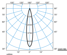
YNSx2LY 7x65 L-SP 01/05 10-940 DD 01 (LEO2)
