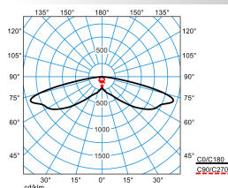
Publisca P2-SB3L/800-730 2G1S TX047920 DIN 5040: A30 UTE: 1,00 l DLOR: 100 % ULOR: 0 % CEN Flux Code: 31 65 93 100 100
