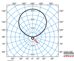
Luceos S G3 PAW-IL 170-8TW ETDS KL 01 (DSU)
