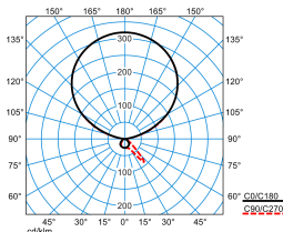
Luceos S G3 PAW-IL 170-8TW ETDS KL 01 (DCW)
