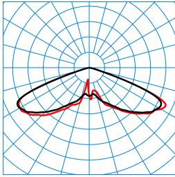
Publisca P2-RB6L/2200-740 3G1S TX047822 ■ C0 - C180 ■ C90 - C270 DIN 5040: A20 UTE: 1,00 J DLOR: 100 % ULOR: 0 % CEN Flux Code: 20 57 98 100 100
