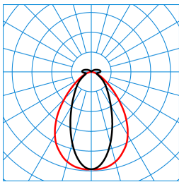
TugraHE 18 PN 100-840 ET IP69K 23 TX425227
