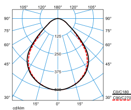
Opendo D2-L PW19 20-47/5/ML-830 ET 01 (2900lm)
