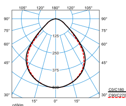
Opendo D2-L PW19 20-47/5/ML-830 ET 01 (3300lm)
