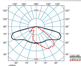
LnPlus 60-AB7L-SLR3/24000-730 18G1 ET (CLO initial value)
