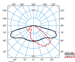
LnPlus 60-AB7L-SLR3/24000-730 18G1 ET (CLO end value)
