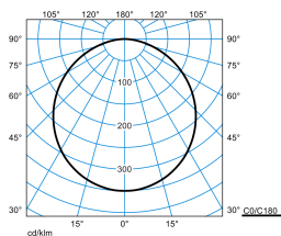
Olisq RWD2 DW 40-830 ETBLE +DMM IP54 PC + Olisq RWD2 ZVF 05
