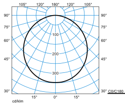
Olisq RWD2 DW 40-830 ETBLE +DMM IP54 PC + Olisq RWD2 ZDR 1/1 01
