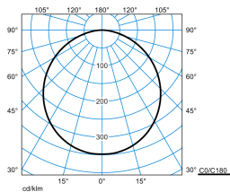
Olisq RWD2 DW 40-830 ETBLE +DMM IP54 PC + Olisq RWD2 ZDR 1/1 05
