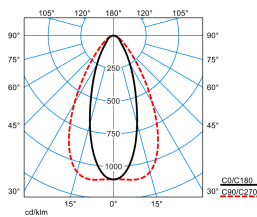
7651IP MironaF T 130-840ETDD L150 01 (LEO2)
