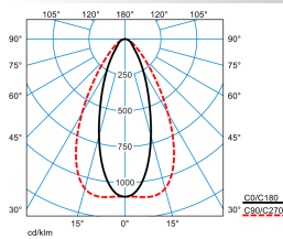
7651IP MironaF T 130-840ETDD L150 01 (LEO1)
