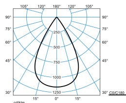
Mirona Fit R LN 150-840 ETDD + REF PC
