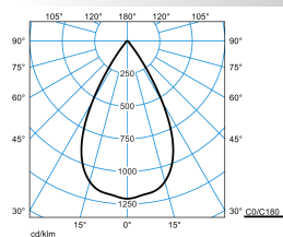
Mirona Fit R LN 150-840 ETDD
