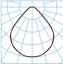
Belviso C2 625 CDP LED3900nw ET 01 TX773249
