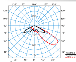
LnPlus 70-AM19L-LR/62000-740 48G1 ET (CLO initial value)
