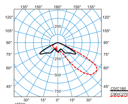
LnPlus 70-AM19L-LR/62000-740 48G1 ET (CLO end value)
