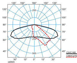
LIQ 50N-AB2L-LR/1350-740 2G1 ET (CLO end value) TX777355
