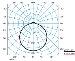
Olisq QWD2 DW 20-840 ET HFS IK
