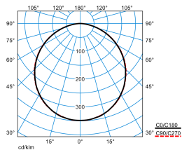
Olisq QWD2 DW 20-840 ET HFS IK + Olisq QWD2 ZDR 1/1 01
