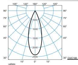
7651 Lentyp L-FL 40-830 M33 ET 01 (225)
