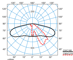
Publisca P1-AB2L-LR/1800-730 2G1S ET (CLO initial value)
