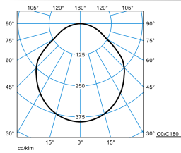
Onplana D11 OTA25 5000-830 ET 01 TX772039
