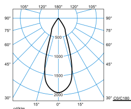
E-Line PRO 78 BV G2 RF-FL 50-830 M33 ETDD 05 Blank
