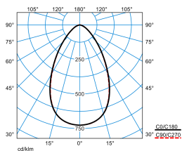
E-Line PRO 78IP50 MironaF TB 270-840 ET L225 01 01 (LEO2)
