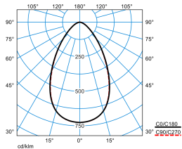
E-Line PRO 78IP50 MironaF TB 270-840 ET L225 01 01 IP50 (LEO1)
