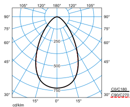
E-Line PRO 78IP50 MironaF TB 270-840 ET L225 01 01 (LEO1)
