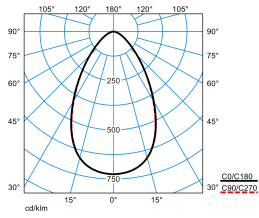
E-Line PRO 78IP50 MironaF TB 270-840 ET L225 01 01 IP50 (LEO3)
