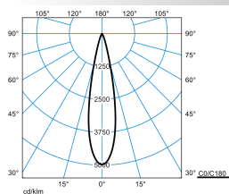
E-Line PRO 78 Lentyp L-SP 30-830 M33 ET 03
