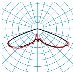
Publisca P2-RB6L-LRA/2000-740 3G1S ET (CLO end value) TX300590 ■ C0 - C180 ■ C90 - C270 DIN 5040: A20 UTE: 1,00 J DLOR: 100 % ULOR: 0 % CEN Flux Code: 20 57 98 100 100
