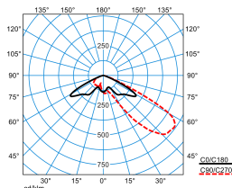
LnPlus 70-AM19L-SLR2/42000-740 36G1 ET (CLO end value)
